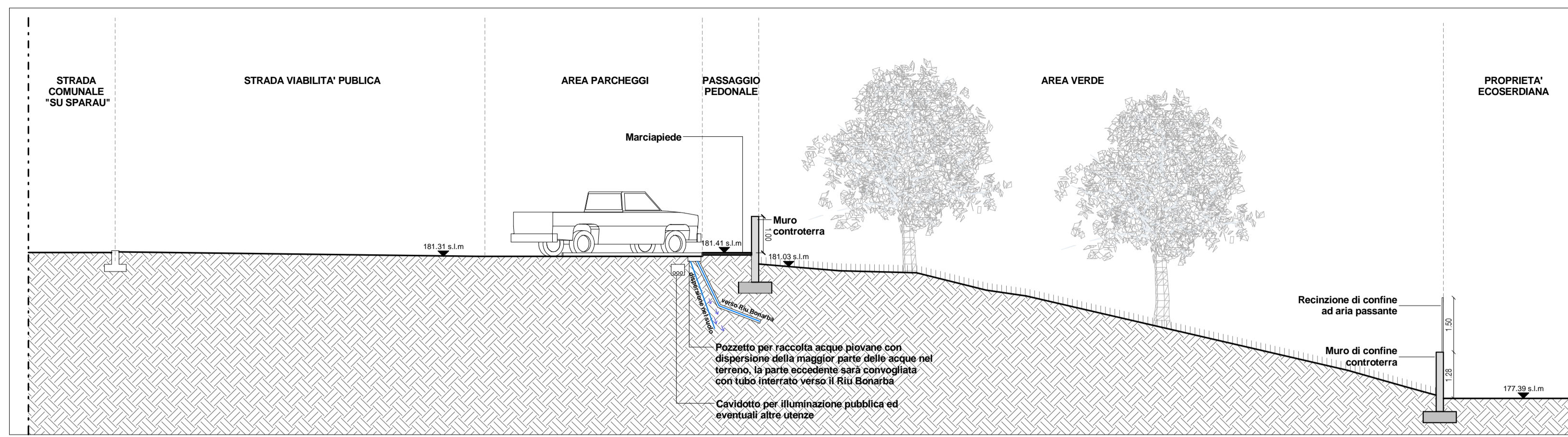
SEZIONE TIPO_A-A
